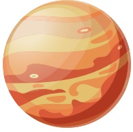
Venus
