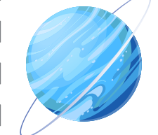
Uranus
